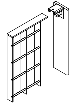
SQUADRETTA TELESCOPICA RETTILINEA
