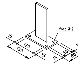
PIANTANA -80x8 lg. 2595 (da tassellare) kg/cad zn. 15,1 DIMENSIONE PIASTRA 150x80x8
