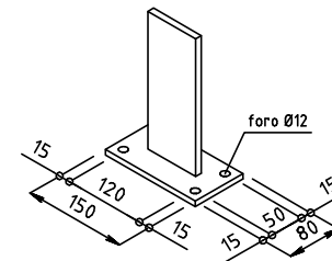
PIANTANA -80x8 lg. 2199 (da tassellare) kg/cad zn. 12,9 DIMENSIONE PIASTRA 150x80x8
