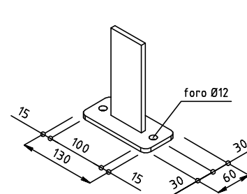
PIANTANA -60x7 lg. 1539 (da tassellare) kg/cad zn. 6,1 DIMENSIONE PIASTRA 130x60x7
