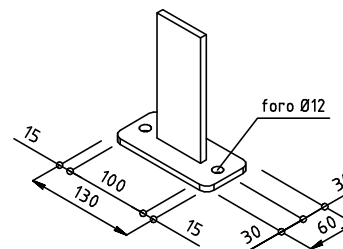
PIANTANA -60x7 lg. 1407 (da tassellare) kg/cad zn. 5,7 DIMENSIONE PIASTRA 130x60x7
